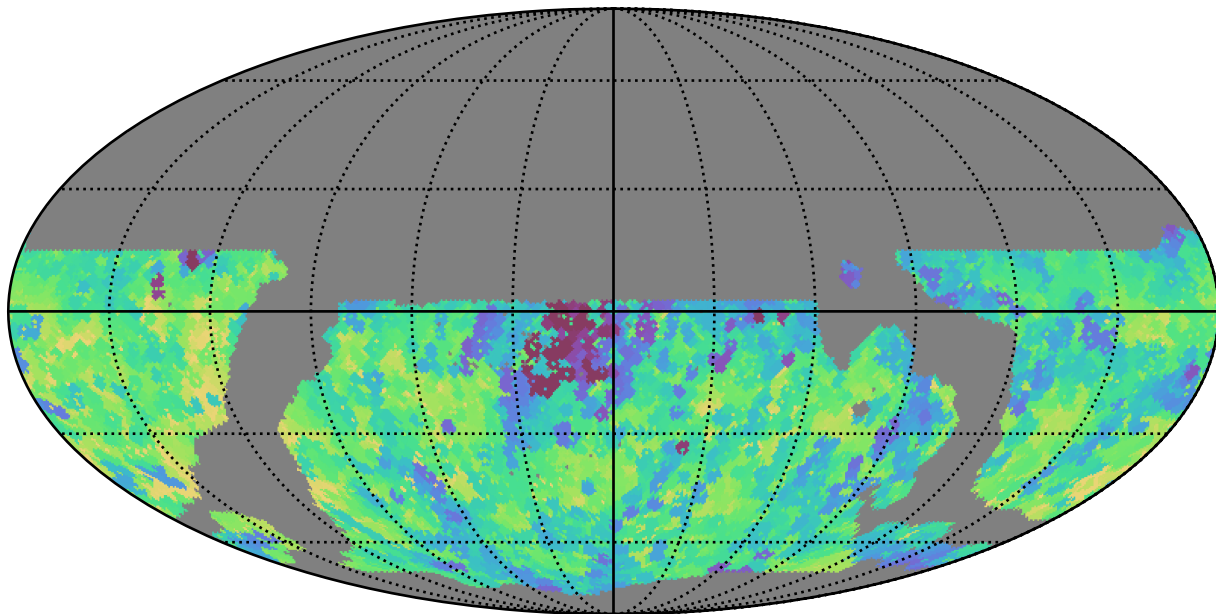
weather_cloudso31v3.4_10yrs WFD r band: Min saturation_mag
