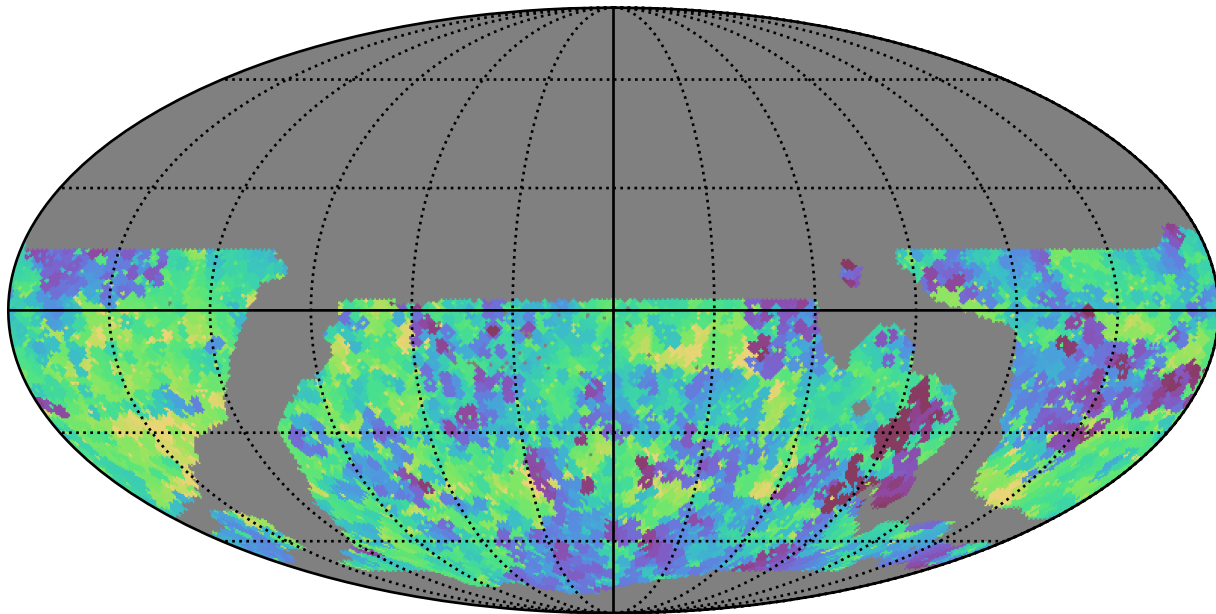
weather_cloudso31v3.4_10yrs WFD g band: Min saturation_mag
