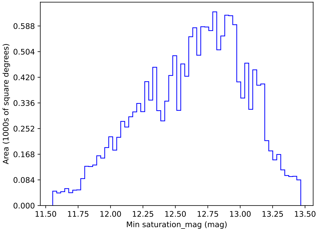
weather_cloudso31v3.4_10yrs WFD g band: Min saturation_mag
