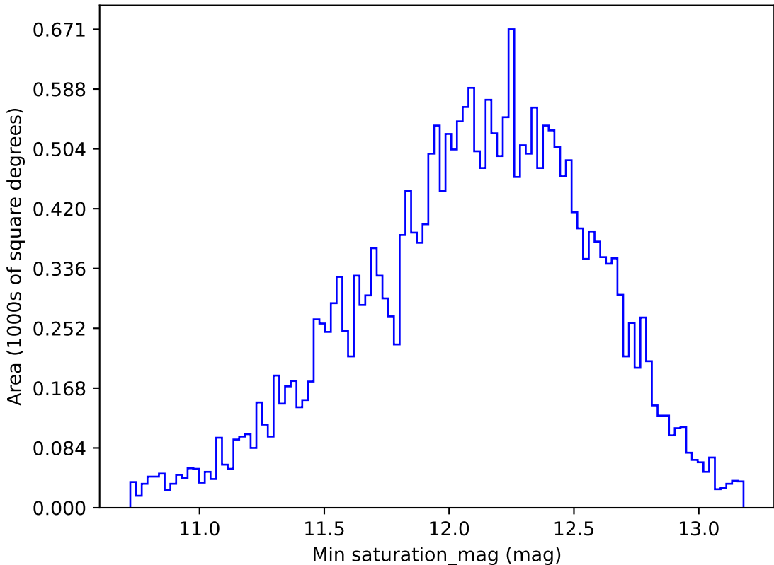
weather_cloudso31v3.4_10yrs All sky z band: Min saturation_mag
