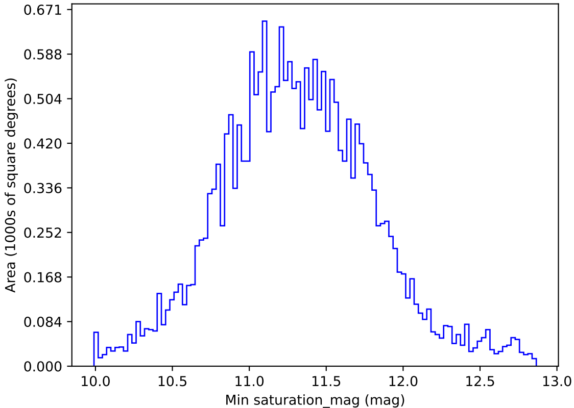
weather_cloudso31v3.4_10yrs All sky u band: Min saturation_mag
