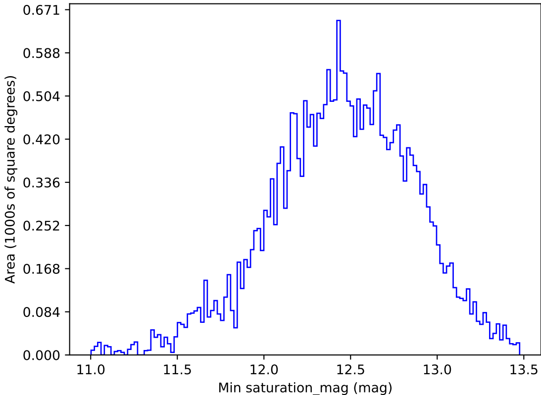
weather_cloudso31v3.4_10yrs All sky r band: Min saturation_mag
