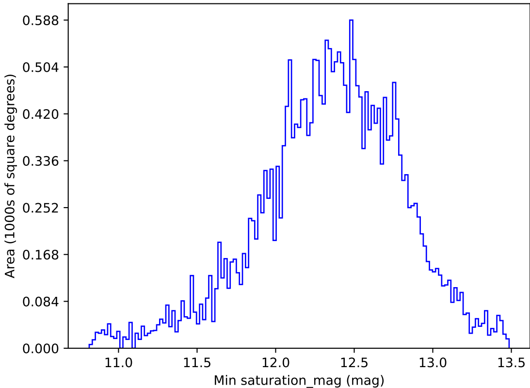
weather_cloudso31v3.4_10yrs All sky i band: Min saturation_mag
