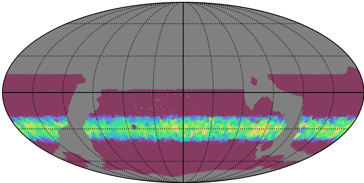
weather_cloudso31v3.4_10yrs WFD z band: Min normairmass
