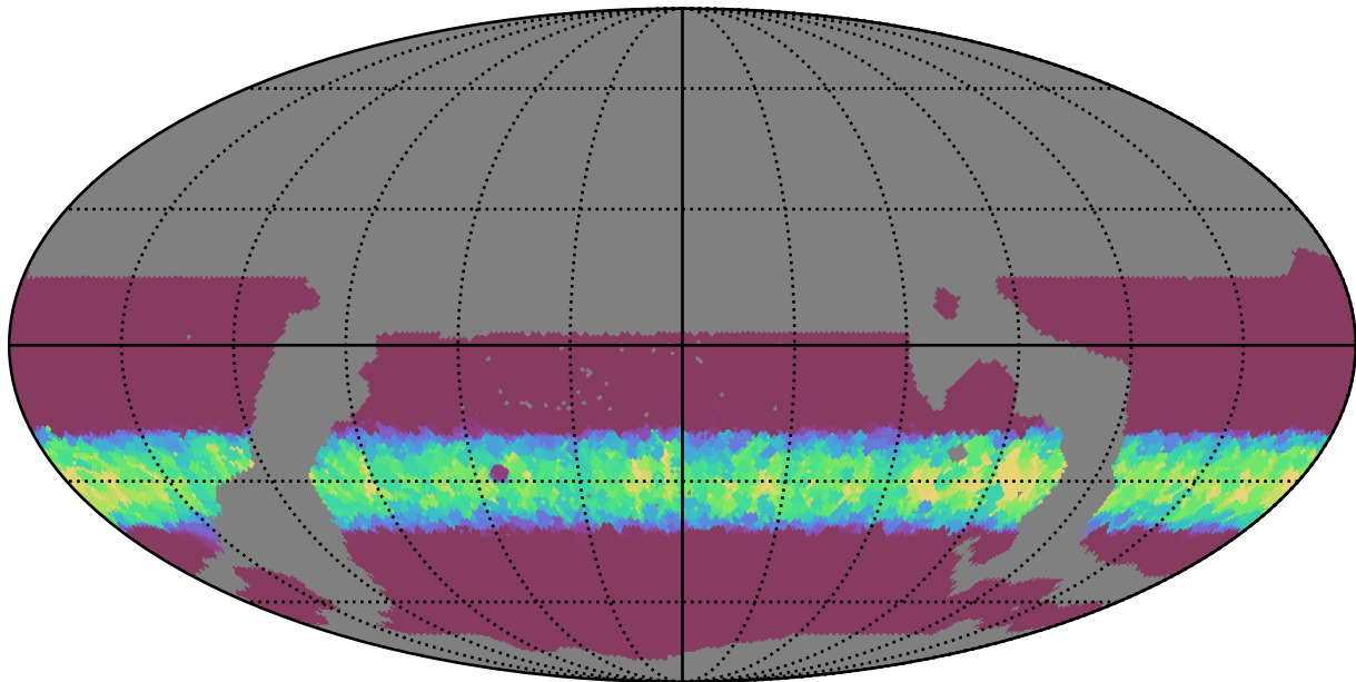
weather_cloudso31v3.4_10yrs WFD y band: Min normairmass
