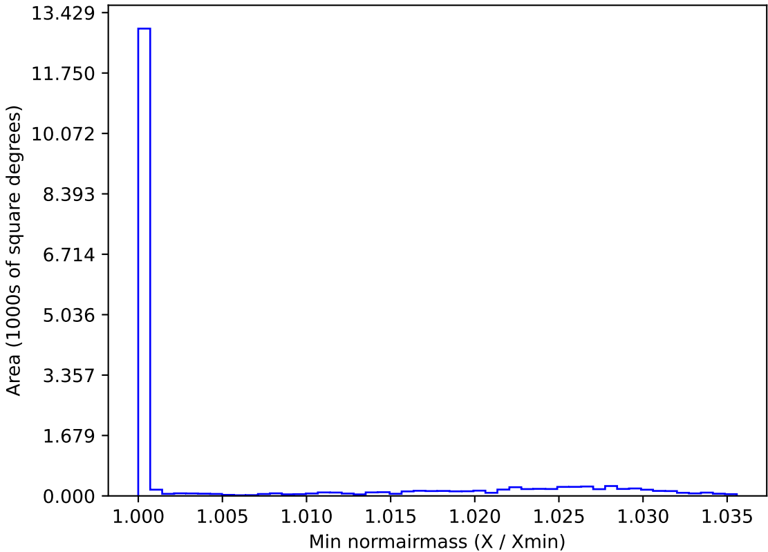
weather_cloudso31v3.4_10yrs WFD i band: Min normairmass
