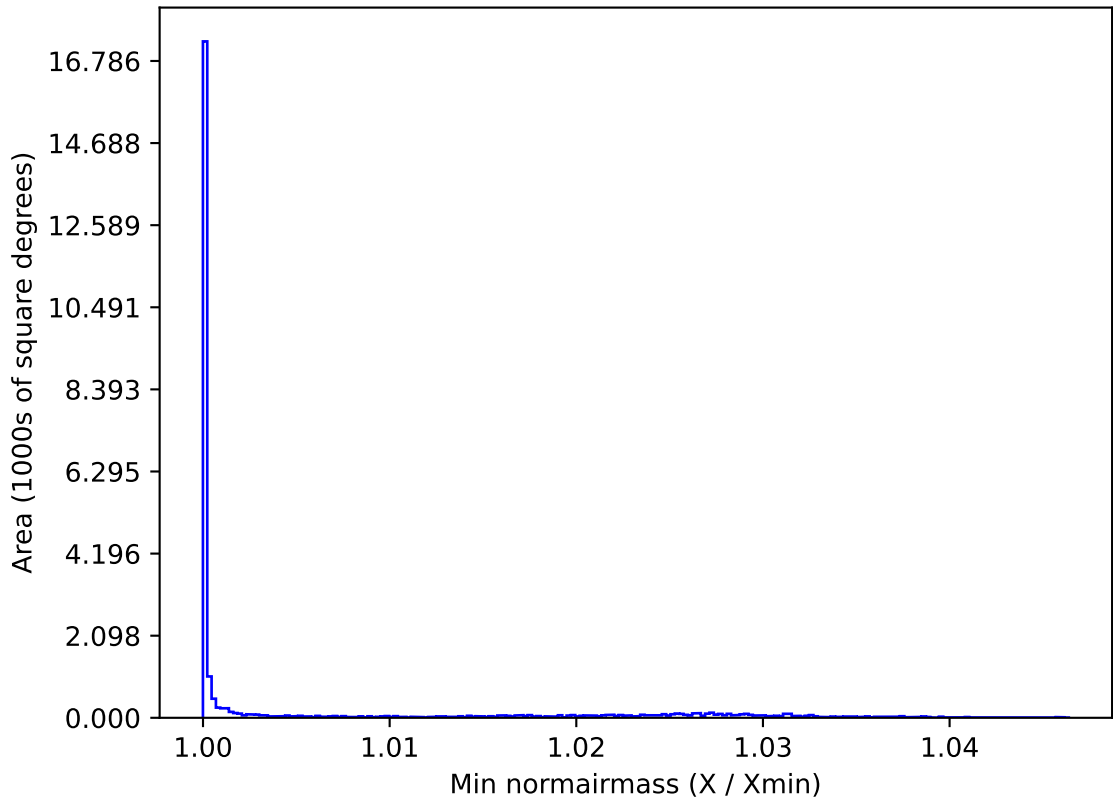
weather_cloudso31v3.4_10yrs All sky z band: Min normairmass
