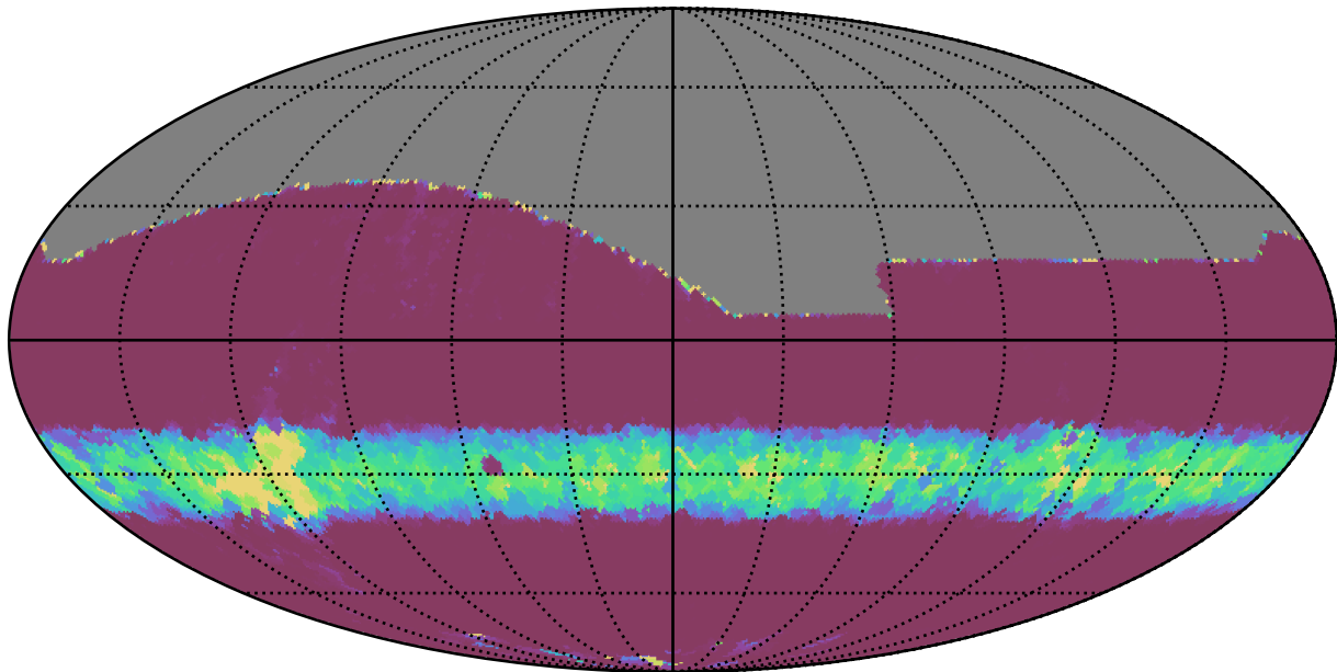
weather_cloudso31v3.4_10yrs All sky i band: Min normairmass
