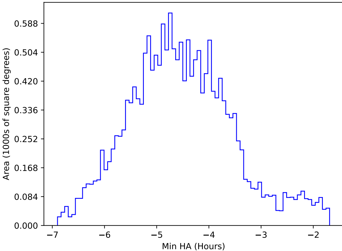
weather_cloudso31v3.4_10yrs WFD z band: Min HA
