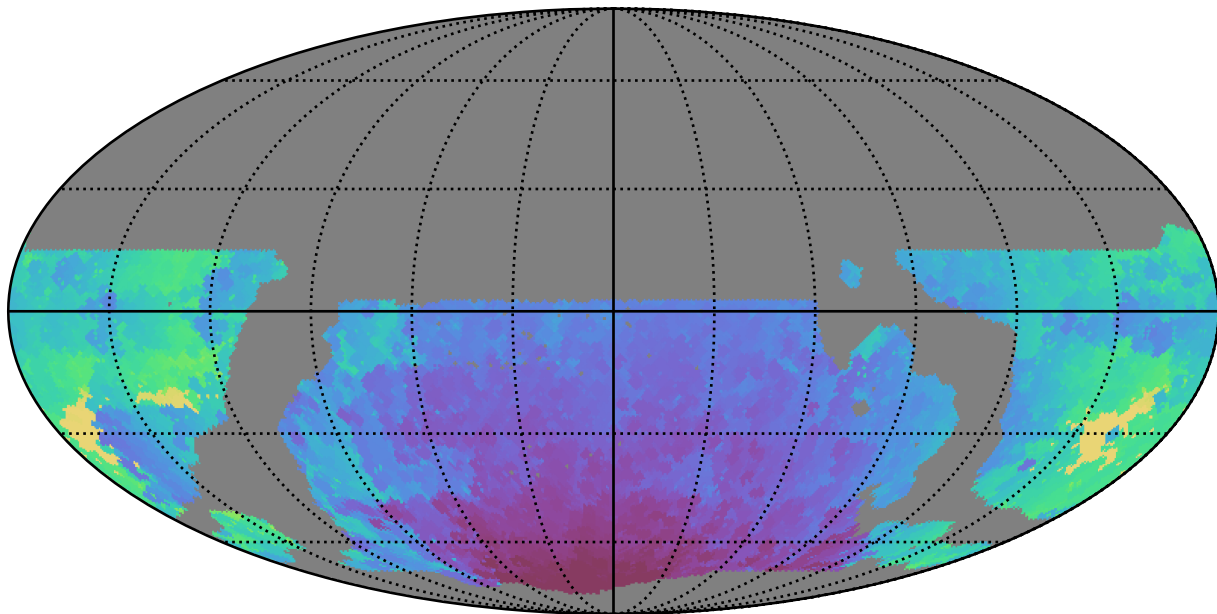
weather_cloudso31v3.4_10yrs WFD y band: Min HA
