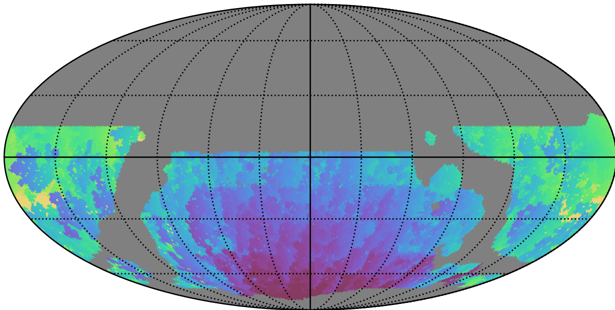
weather_cloudso31v3.4_10yrs WFD u band: Min HA
