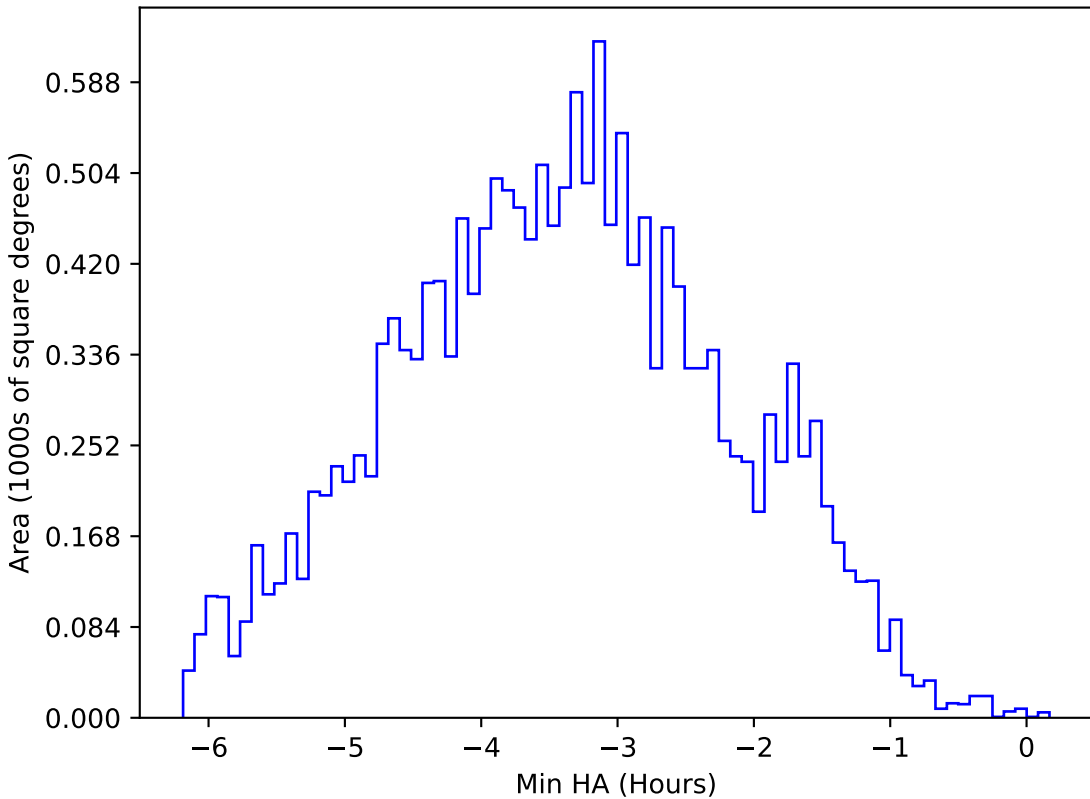
weather_cloudso31v3.4_10yrs WFD u band: Min HA
