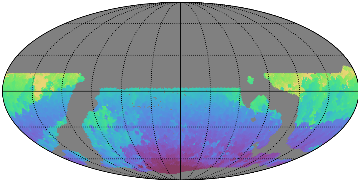
weather_cloudso31v3.4_10yrs WFD r band: Min HA
