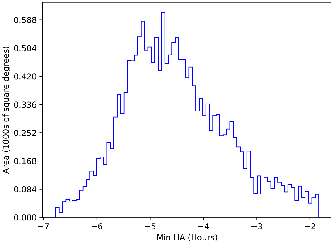
weather_cloudso31v3.4_10yrs WFD r band: Min HA
