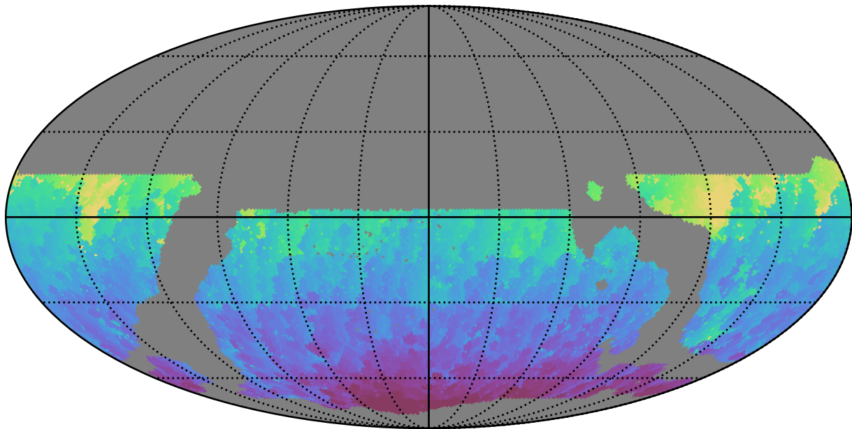
weather_cloudso31v3.4_10yrs WFD g band: Min HA
