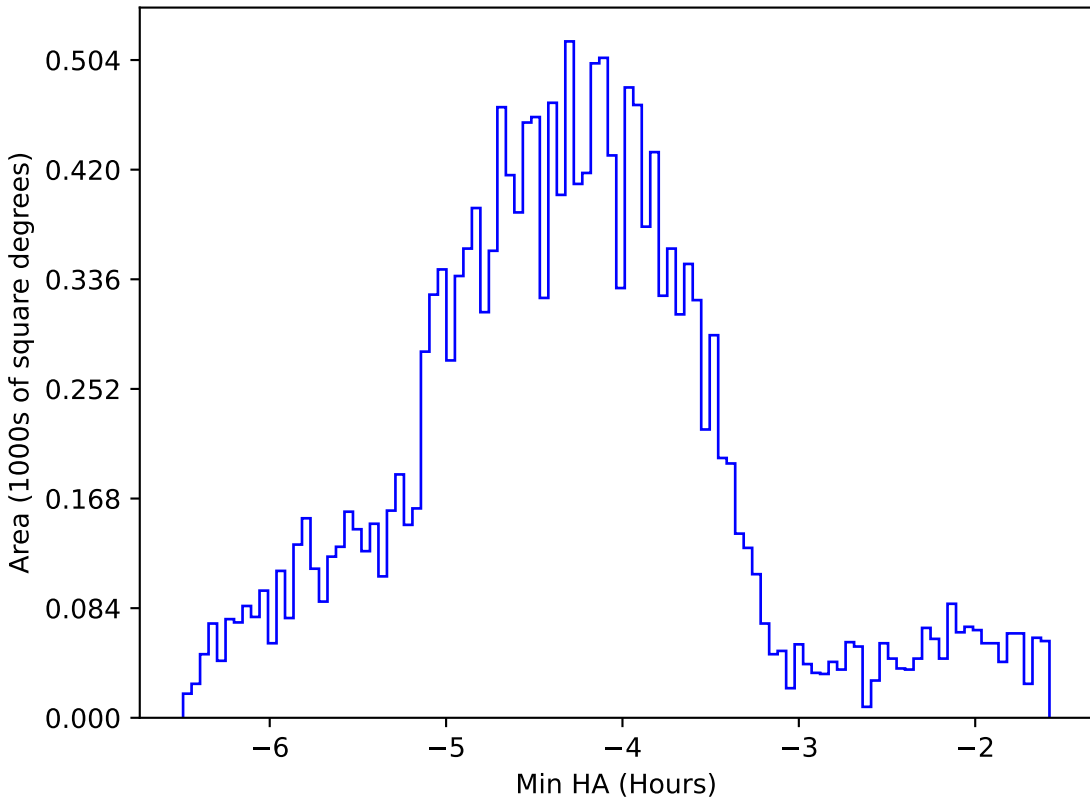
weather_cloudso31v3.4_10yrs WFD g band: Min HA
