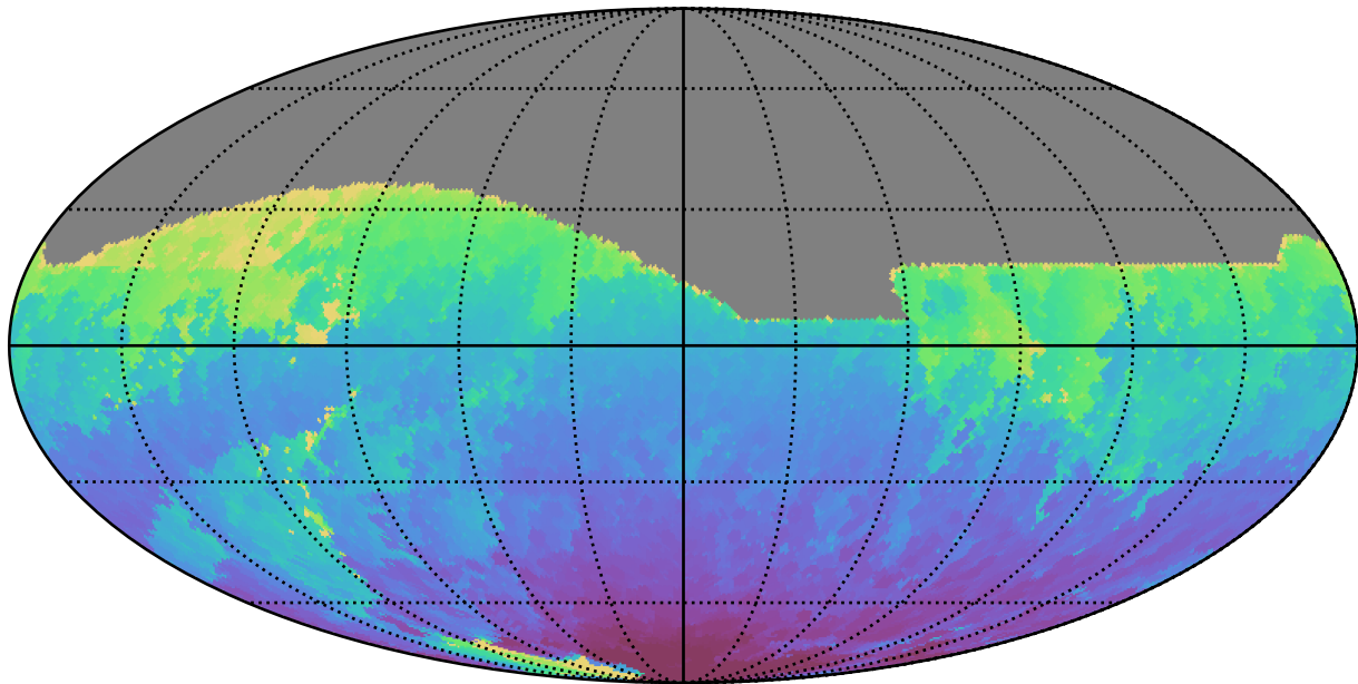
weather_cloudso31v3.4_10yrs All sky z band: Min HA
