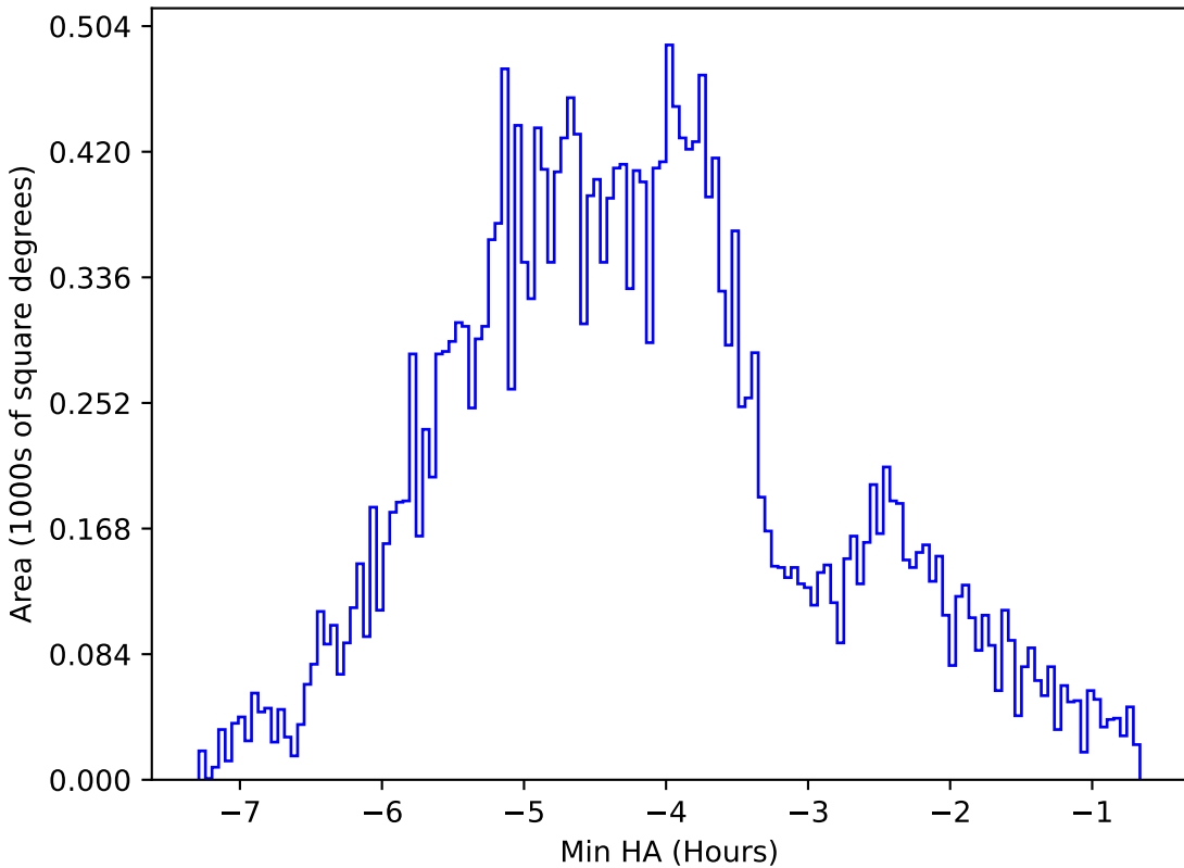
weather_cloudso31v3.4_10yrs All sky z band: Min HA
