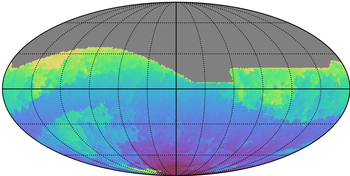
weather_cloudso31v3.4_10yrs All sky r band: Min HA
