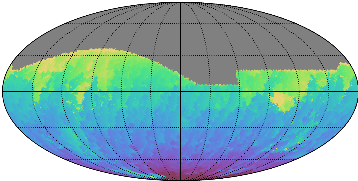
weather_cloudso31v3.4_10yrs All sky g band: Min HA
