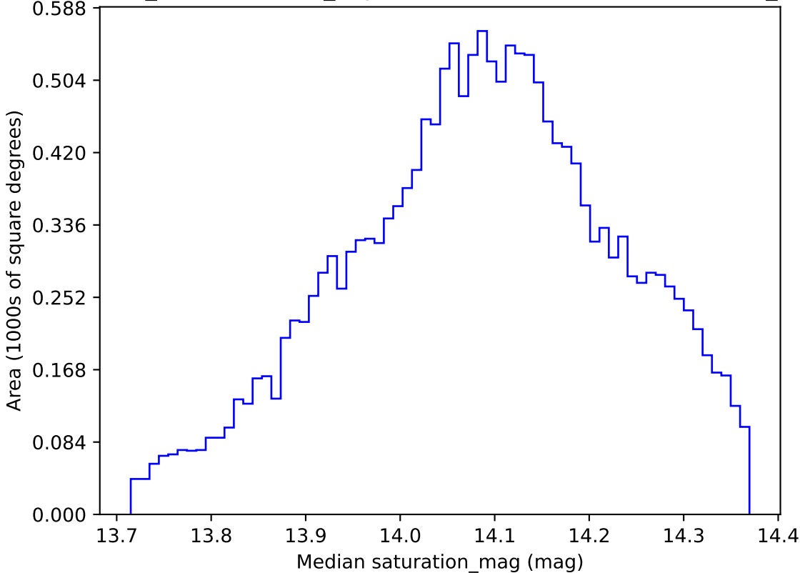
weather_cloudso31v3.4_10yrs WFD z band: Median saturation_mag
