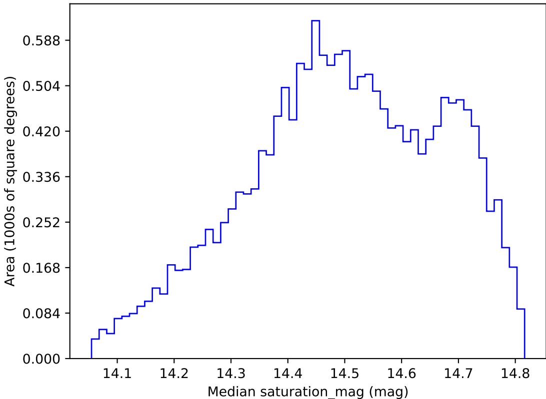
weather_cloudso31v3.4_10yrs WFD i band: Median saturation_mag
