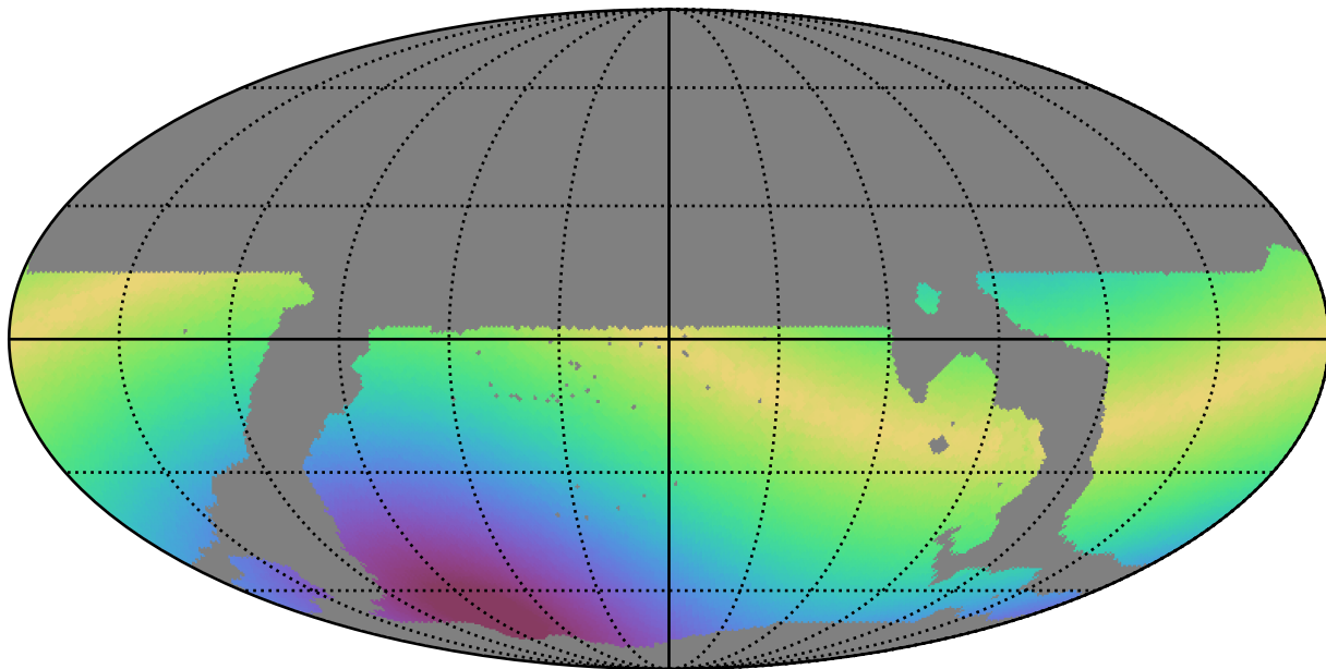
weather_cloudso31v3.4_10yrs WFD y band: Max solarElong
