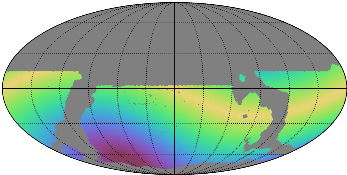
weather_cloudso31v3.4_10yrs WFD i band: Max solarElong
