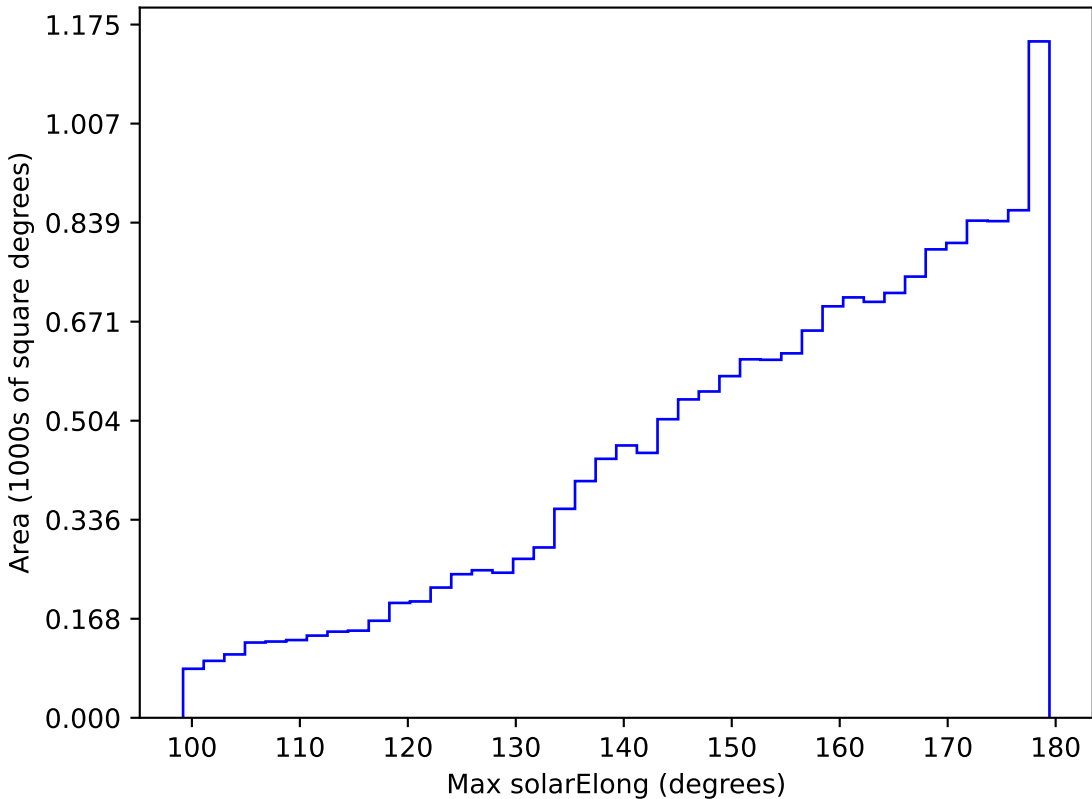
weather_cloudso31v3.4_10yrs WFD i band: Max solarElong
