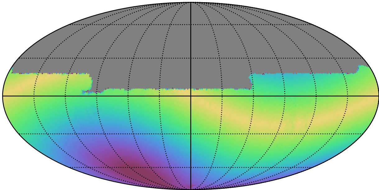
weather_cloudso31v3.4_10yrs All sky y band: Max solarElong
