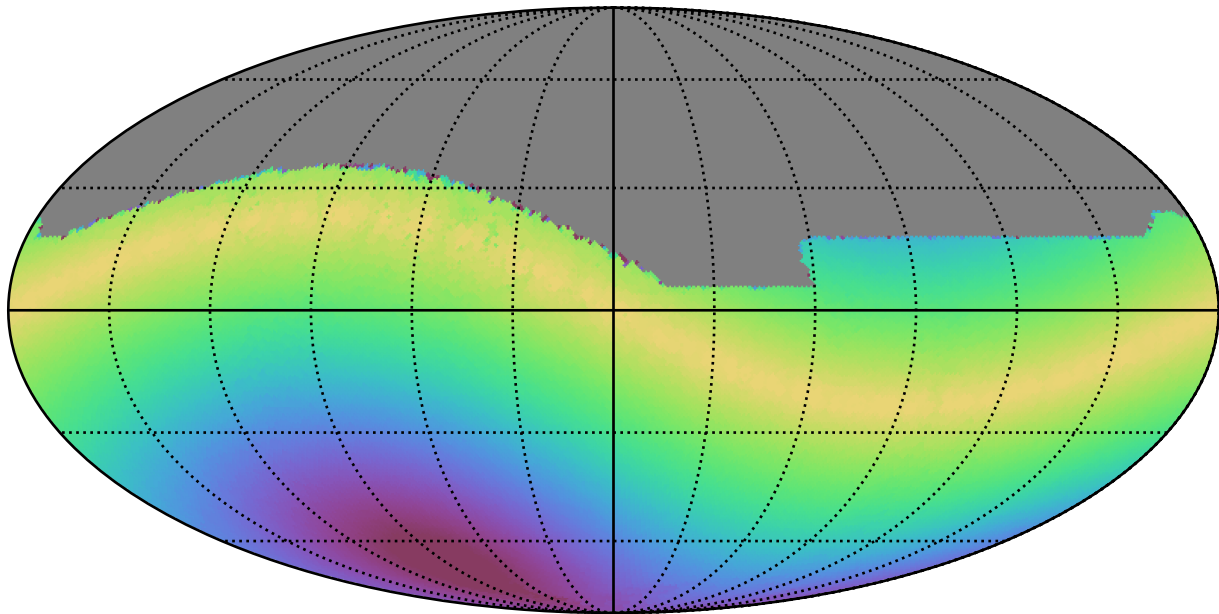
weather_cloudso31v3.4_10yrs All sky i band: Max solarElong
