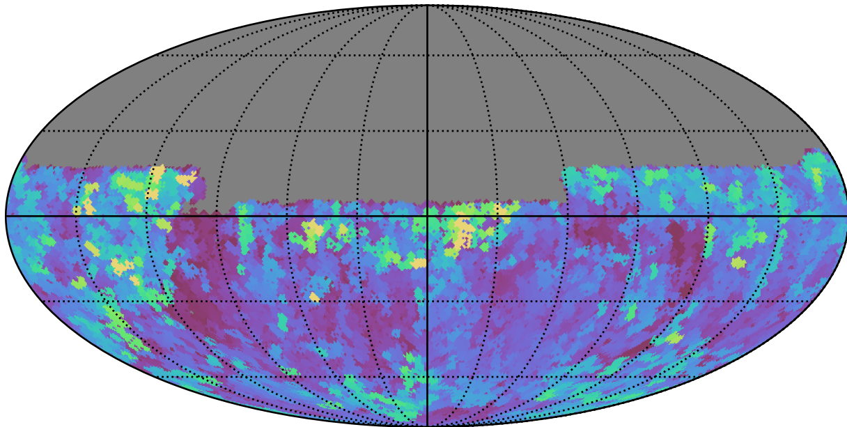
weather_cloudso31v3.4_10yrs Yr 1 y band: Max seeingGeom
