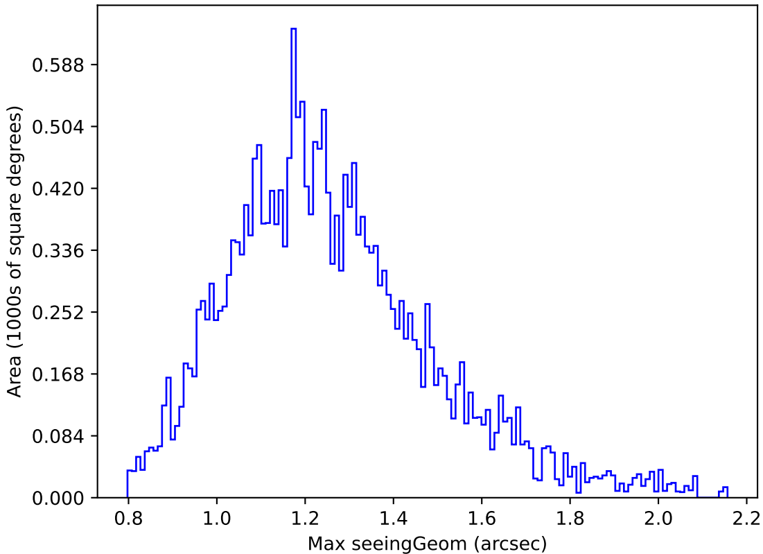
weather_cloudso31v3.4_10yrs Yr 1 y band: Max seeingGeom
