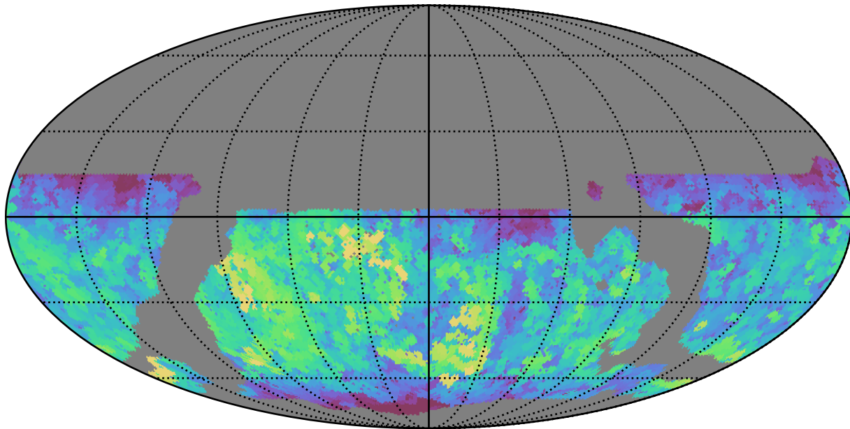
weather_cloudso31v3.4_10yrs WFD z band: Max saturation_mag
