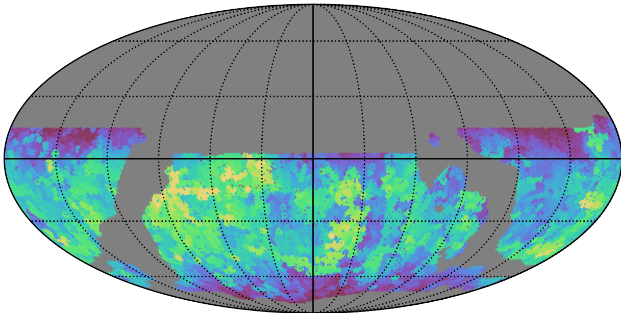
weather_cloudso31v3.4_10yrs WFD y band: Max saturation_mag
