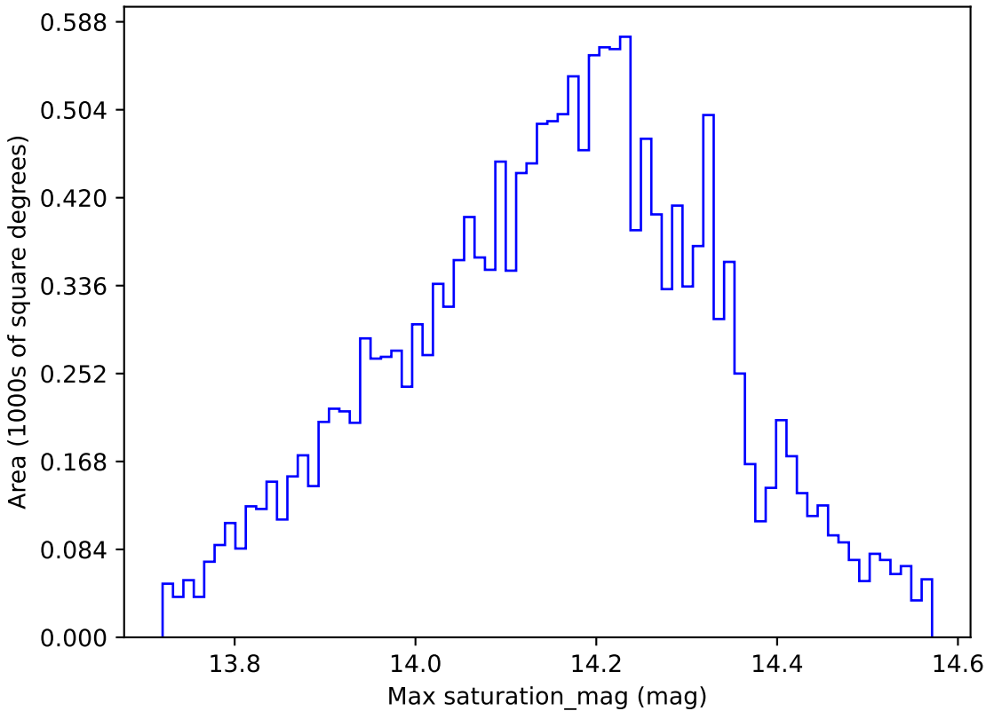
weather_cloudso31v3.4_10yrs WFD y band: Max saturation_mag
