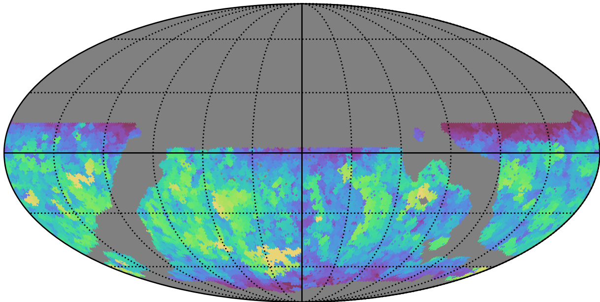
weather_cloudso31v3.4_10yrs WFD r band: Max saturation_mag
