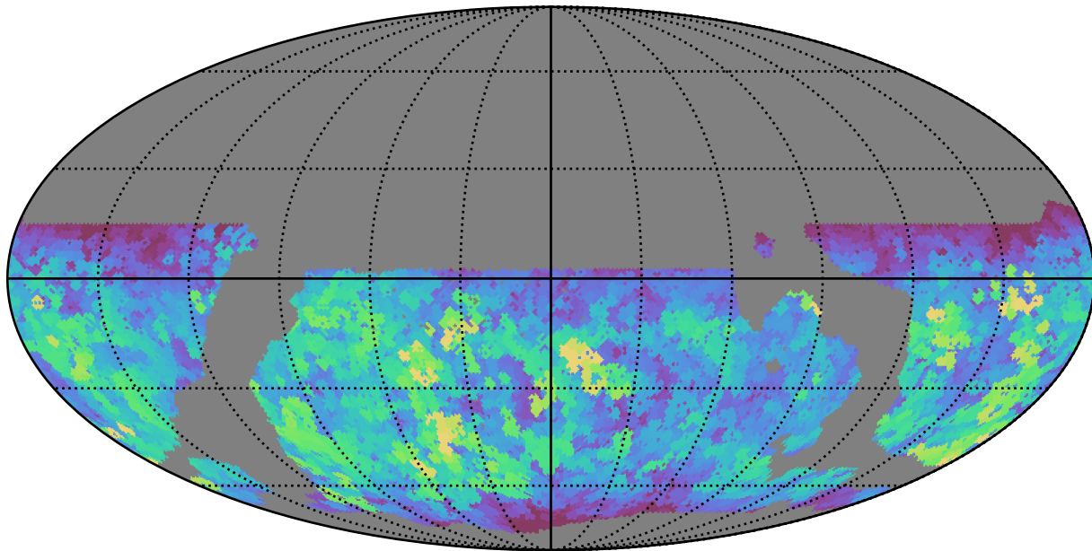
weather_cloudso31v3.4_10yrs WFD i band: Max saturation_mag
