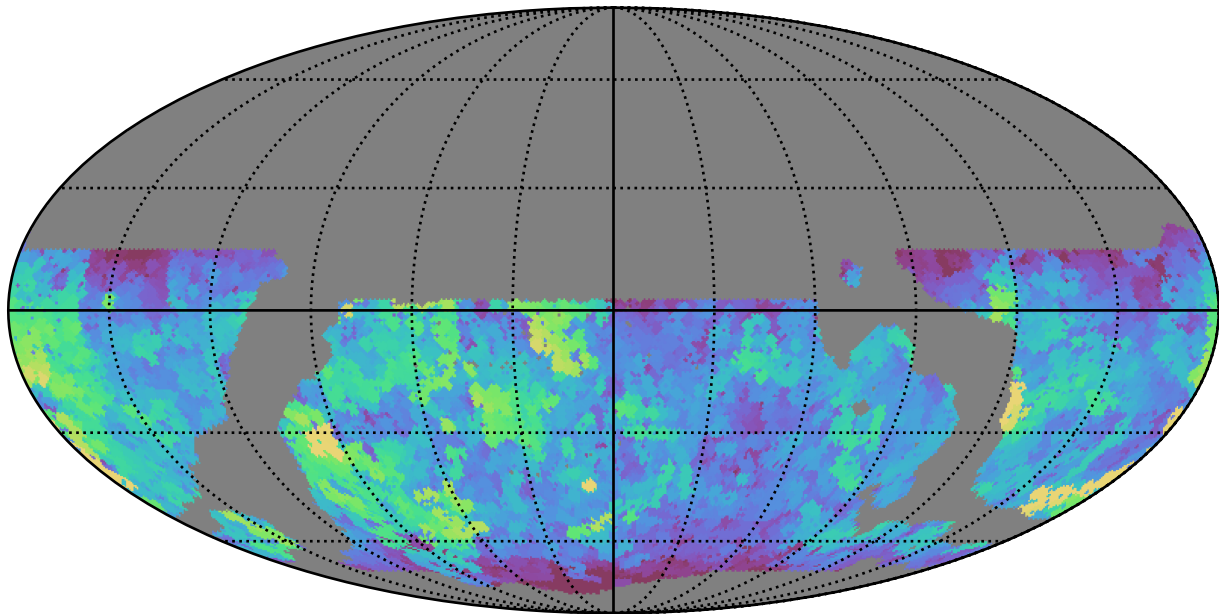
weather_cloudso31v3.4_10yrs WFD g band: Max saturation_mag
