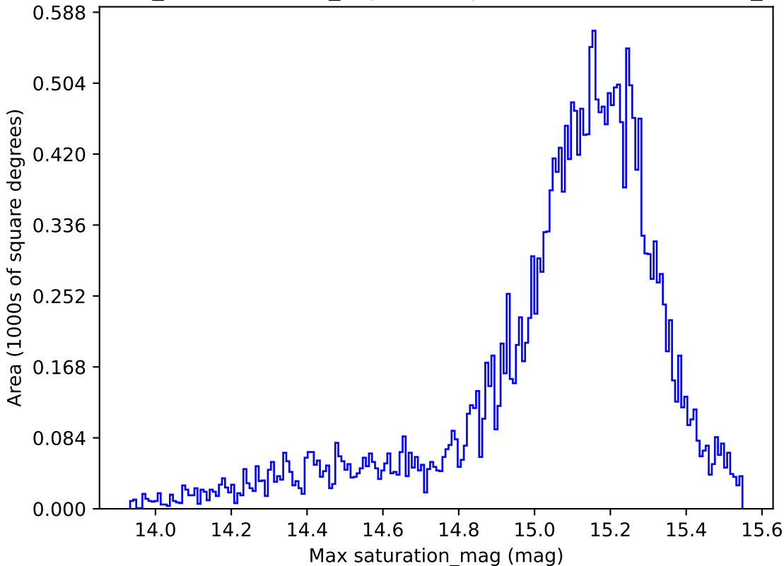
weather_cloudso31v3.4_10yrs All sky z band: Max saturation_mag
