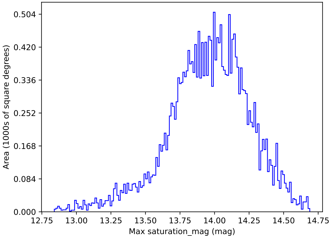
weather_cloudso31v3.4_10yrs All sky u band: Max saturation_mag
