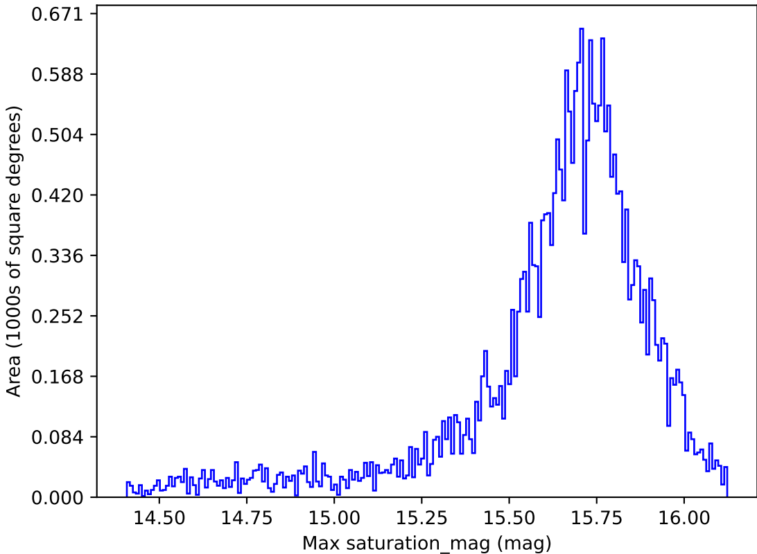
weather_cloudso31v3.4_10yrs All sky r band: Max saturation_mag
