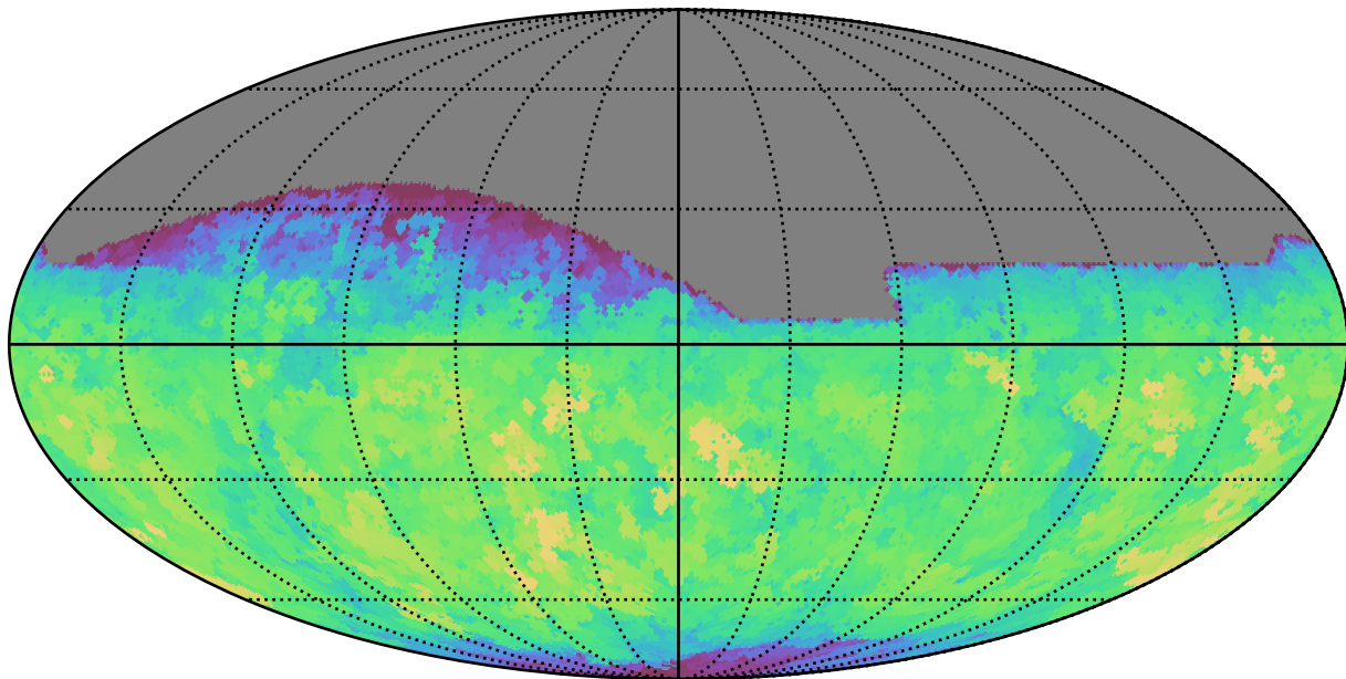
weather_cloudso31v3.4_10yrs All sky i band: Max saturation_mag
