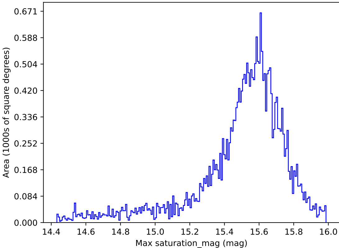
weather_cloudso31v3.4_10yrs All sky i band: Max saturation_mag
