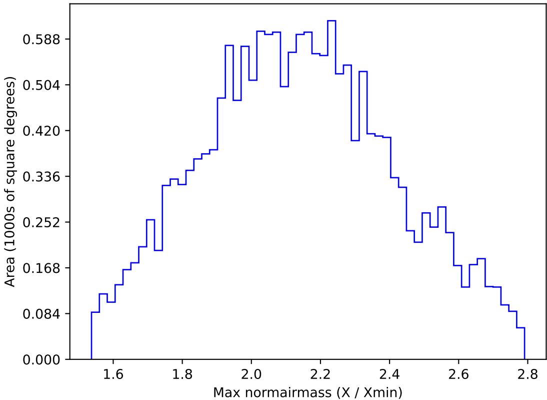
weather_cloudso31v3.4_10yrs WFD y band: Max normairmass
