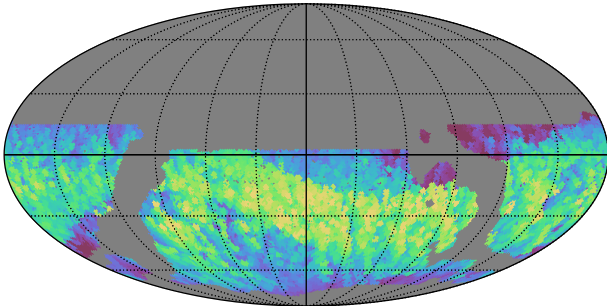
weather_cloudso31v3.4_10yrs WFD i band: Max normairmass
