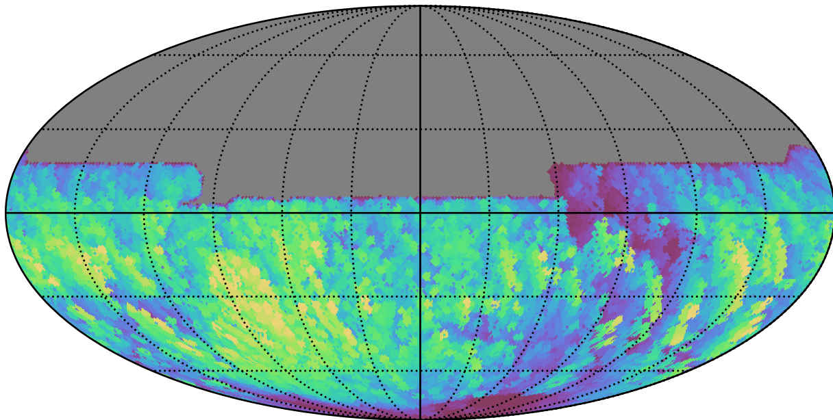
weather_cloudso31v3.4_10yrs All sky y band: Max normairmass
