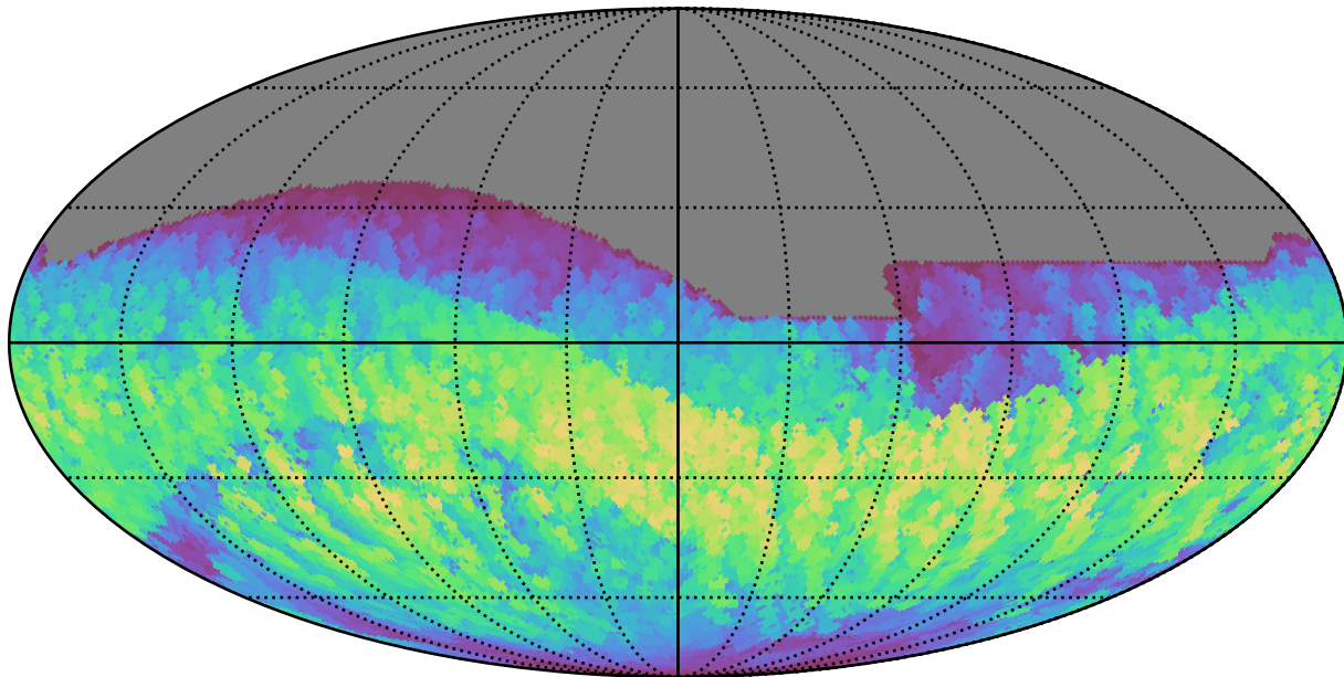
weather_cloudso31v3.4_10yrs All sky i band: Max normairmass
