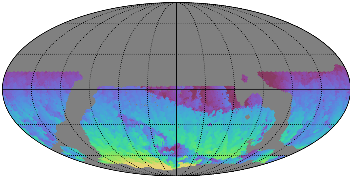
weather_cloudso31v3.4_10yrs WFD z band: Max HA
