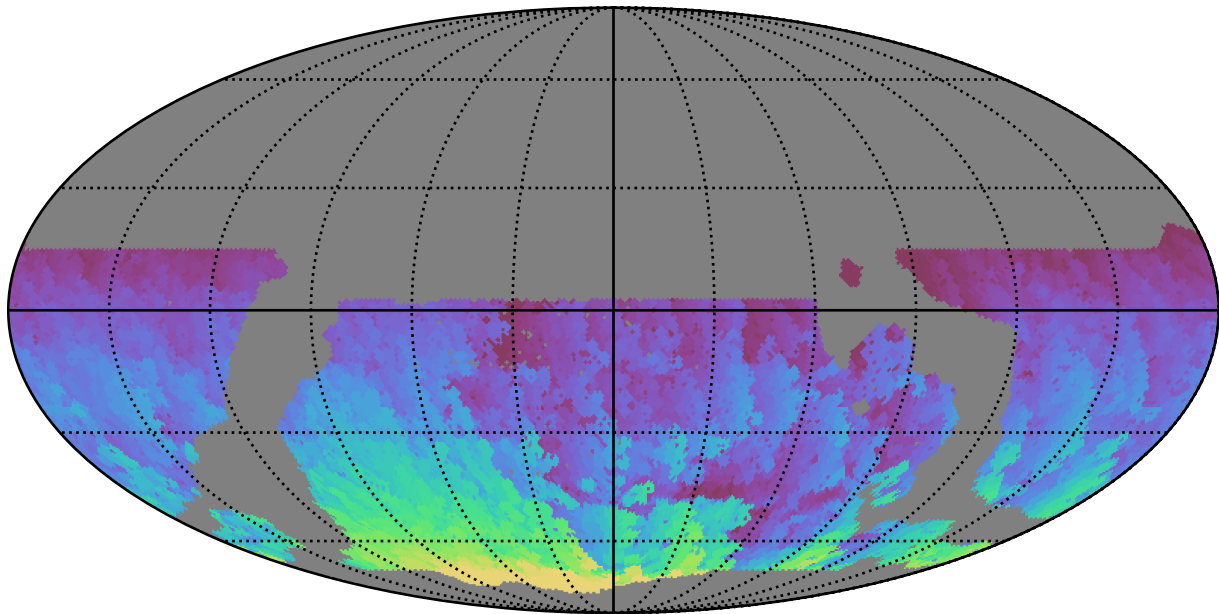
weather_cloudso31v3.4_10yrs WFD y band: Max HA
